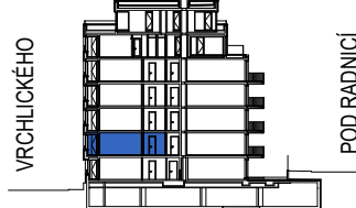
řez budovou
